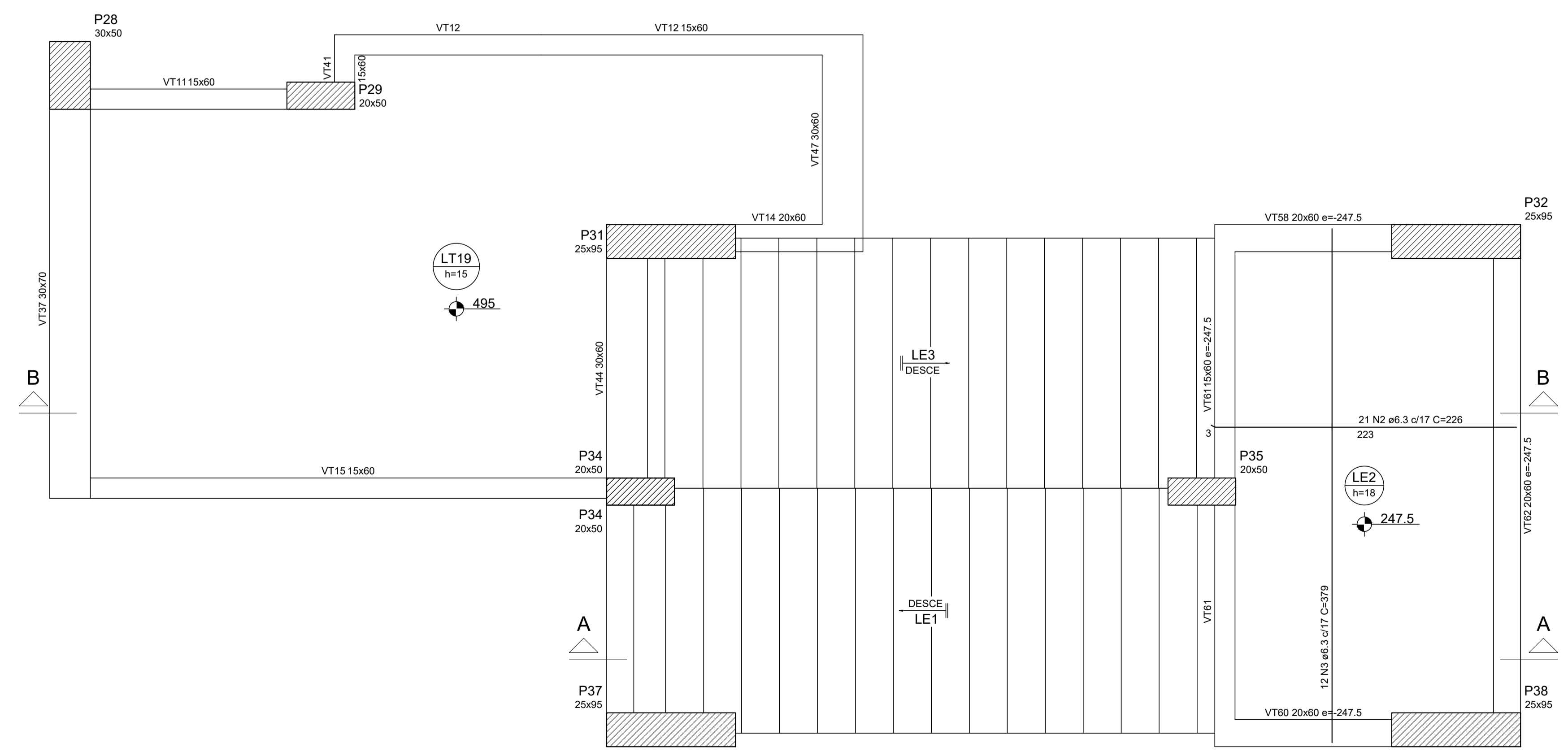
Armação positiva da escada E3 ESC 1:25
