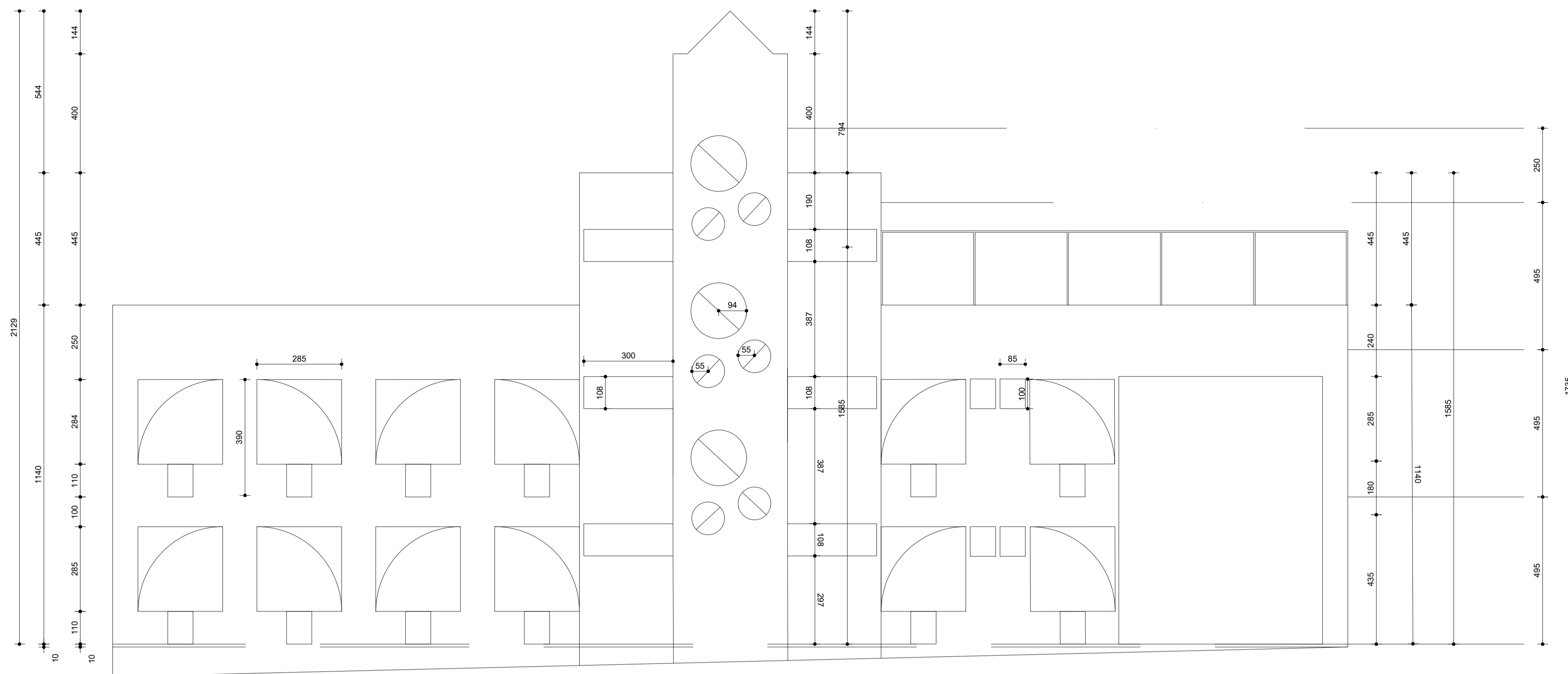
7 Fachada Lateral Escala 1:100
